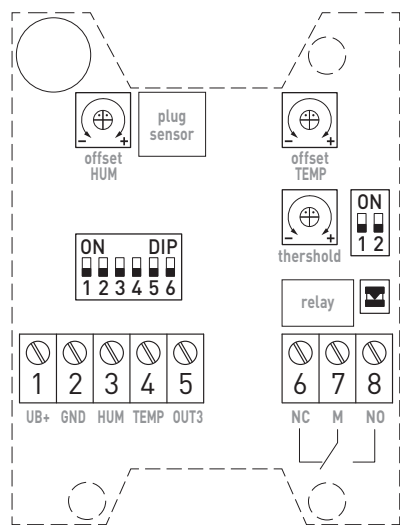
Схема подключения AFTF-45-xx
