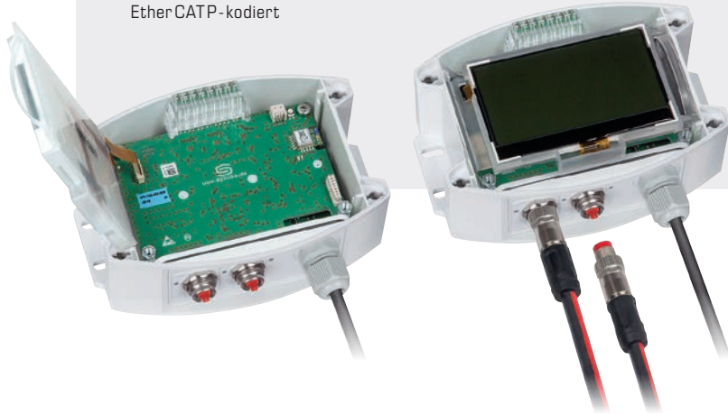
M8-Steckverbinder EtherCATP-kodiert
