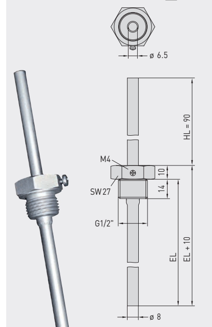
Габаритный чертёж
