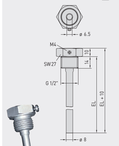
Габаритный чертёж
