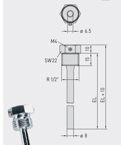
Габаритный чертёж
