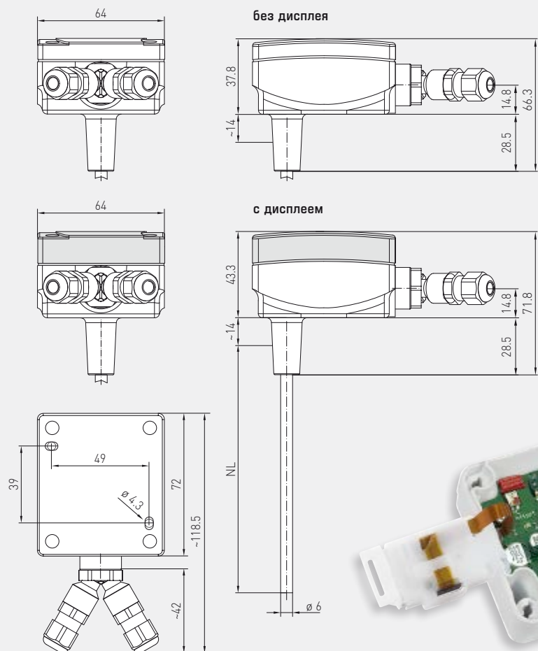
Габаритный чертеж
