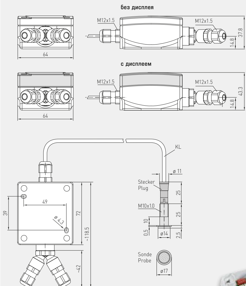
Габаритный чертеж
